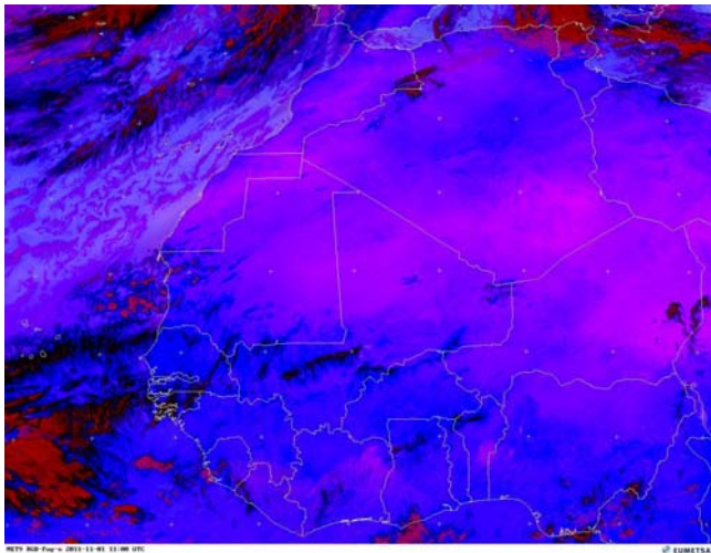
صور الأقمار الصناعية ليوم 01.11.2011 عند الساعة 11:00
